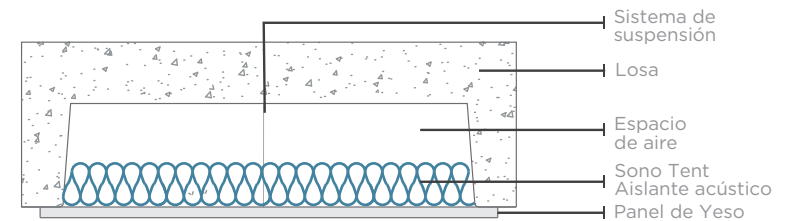
Esquema 2 Aislamiento de 58 STC
