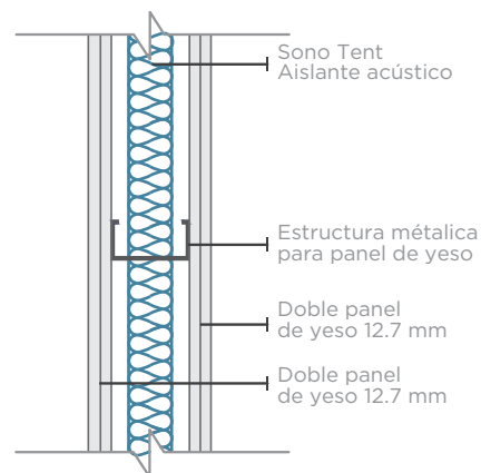
Esquema 2 Absorción de 51 STC
