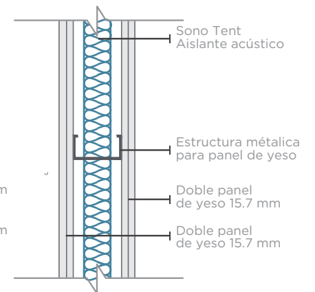
Esquema 4 Absorción de 55 STC
