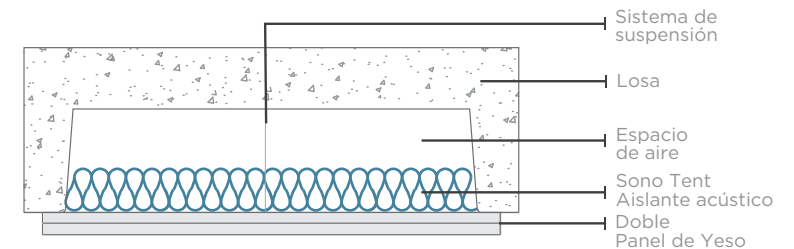
Esquema 2 Aislamiento de 58 STC
