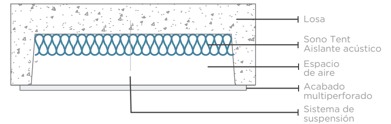
Esquema 1 Absorción de 0.99 NRC
