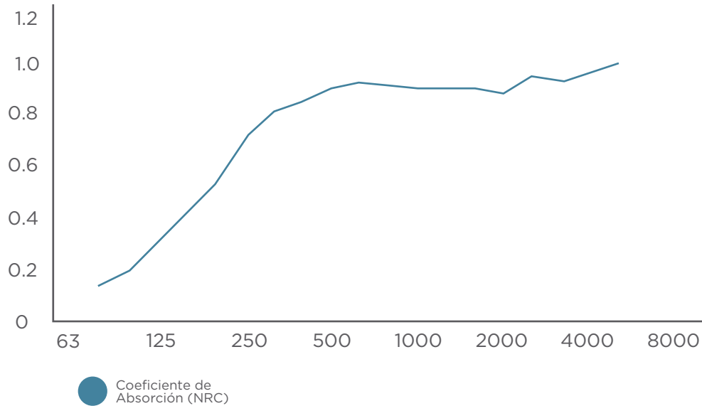
Esquema 1 Absorción de 0.99 NRC
