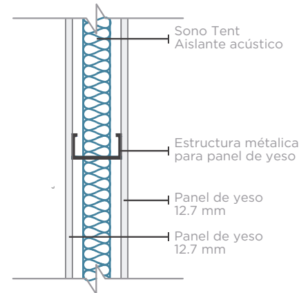
Esquema 1 Aislamiento de 45 STC
