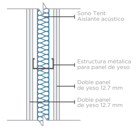
Esquema 2 Absorción de 51 STC
